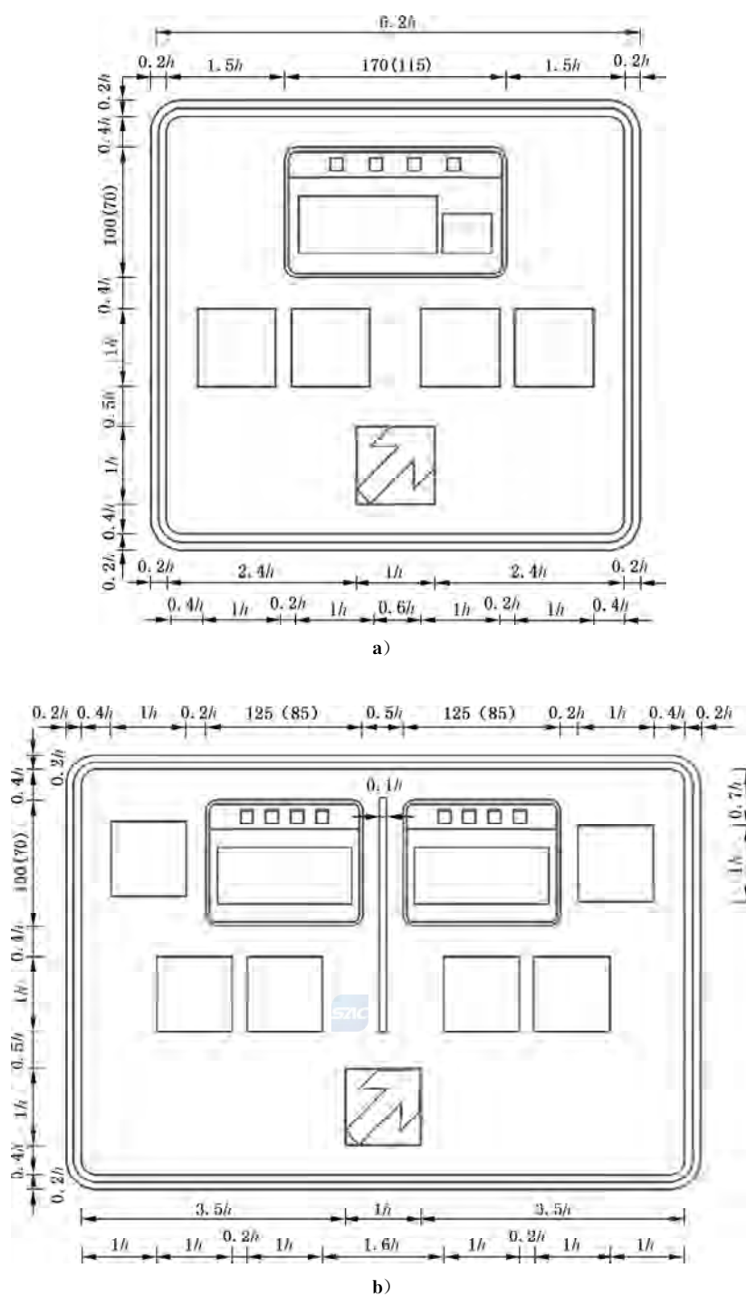
图 E.213 对应路 47 的制作图例
