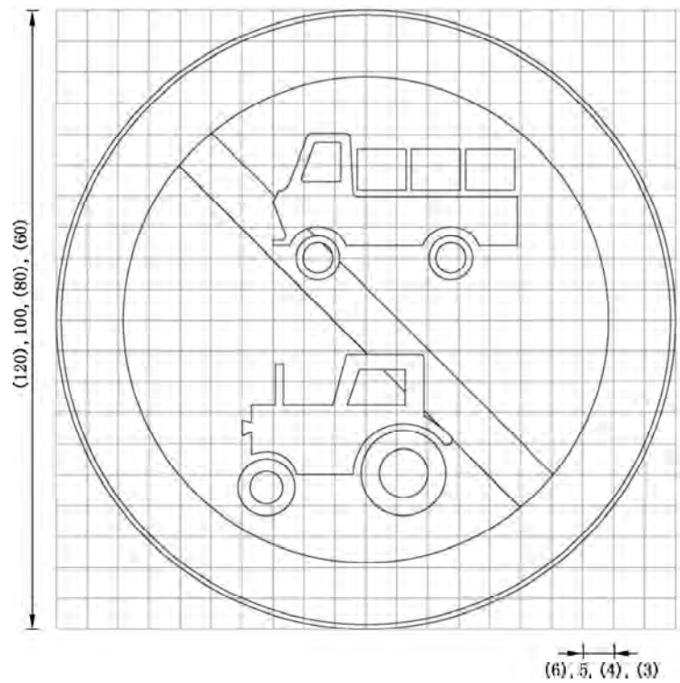
图 E.22 对应禁 22 的制作图例
