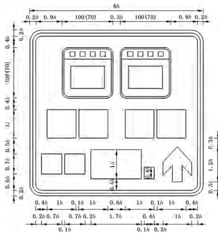
图 E.197 对应路 32 的制作图例
