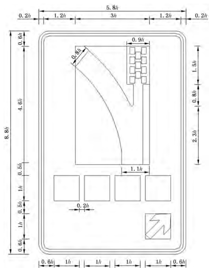
图 E.163 对应警 43-1 的制作图例
