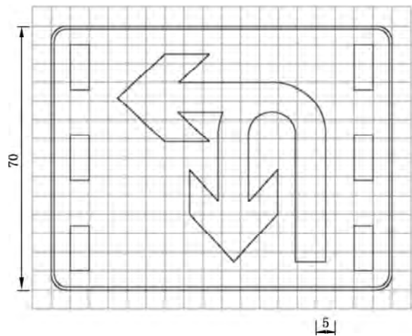
图 E.72 对应示 23 的制作图例
