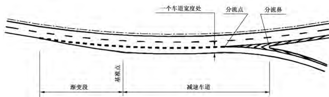
b) 平行式单车道出口
