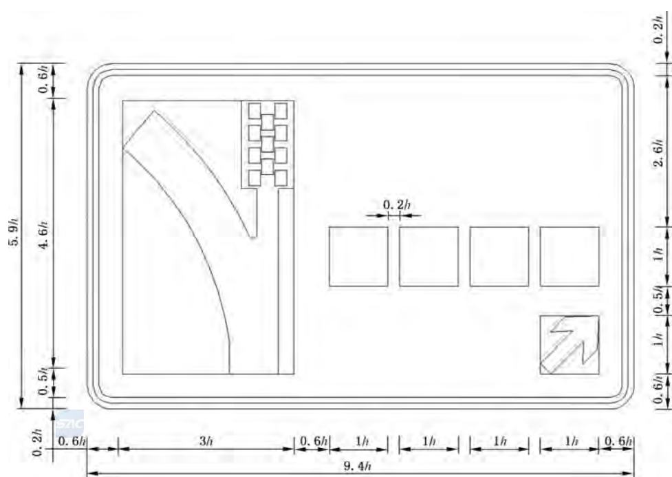
图 E.164 对应警 43-2 的制作图例
