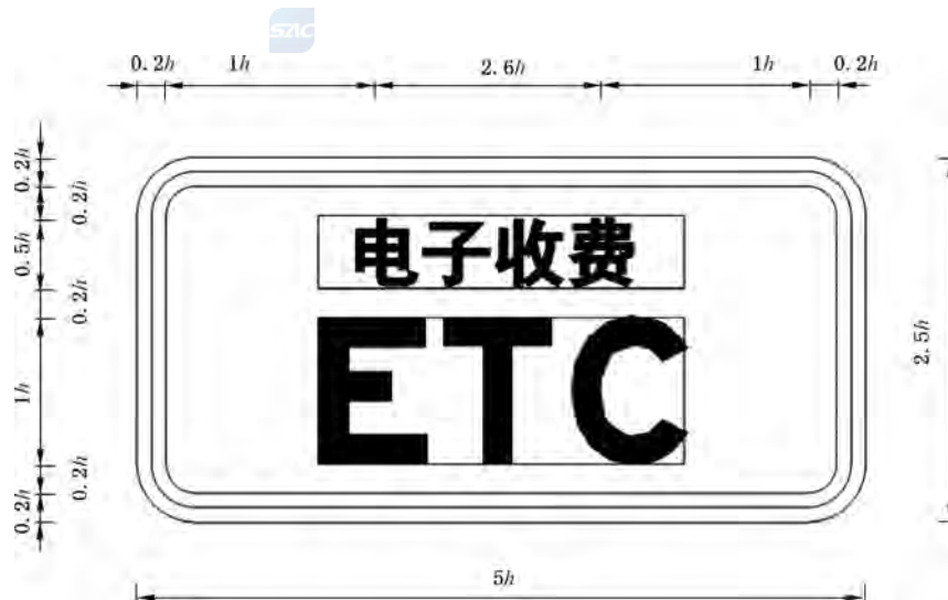
图 E.239 对应路 72 的制作图例
