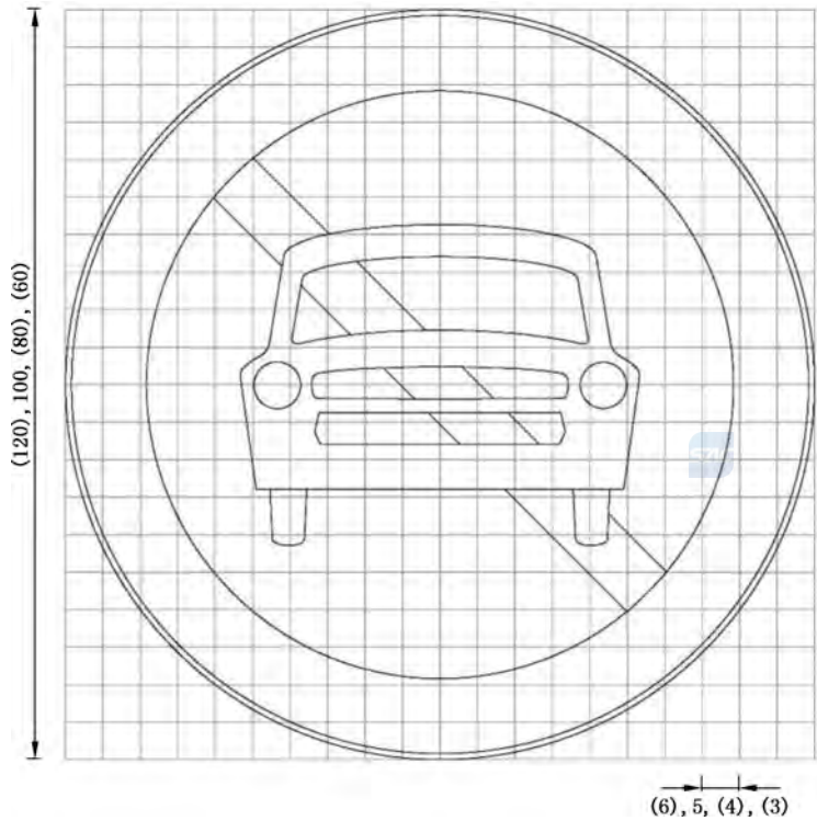
图 E.6 对应禁 6 的制作图例
