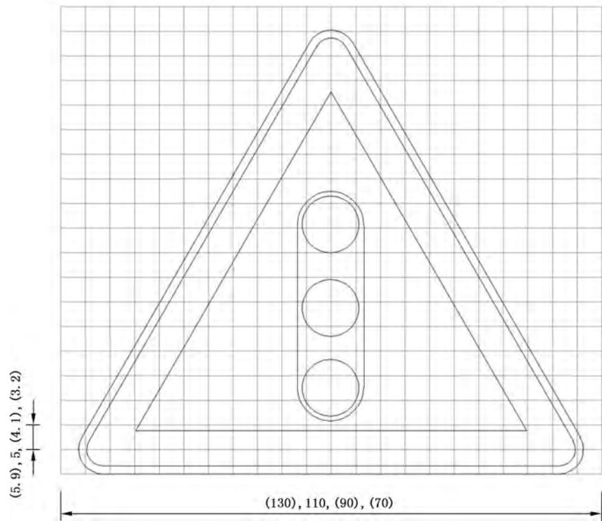
图 E.132 对应警 17 的制作图例
