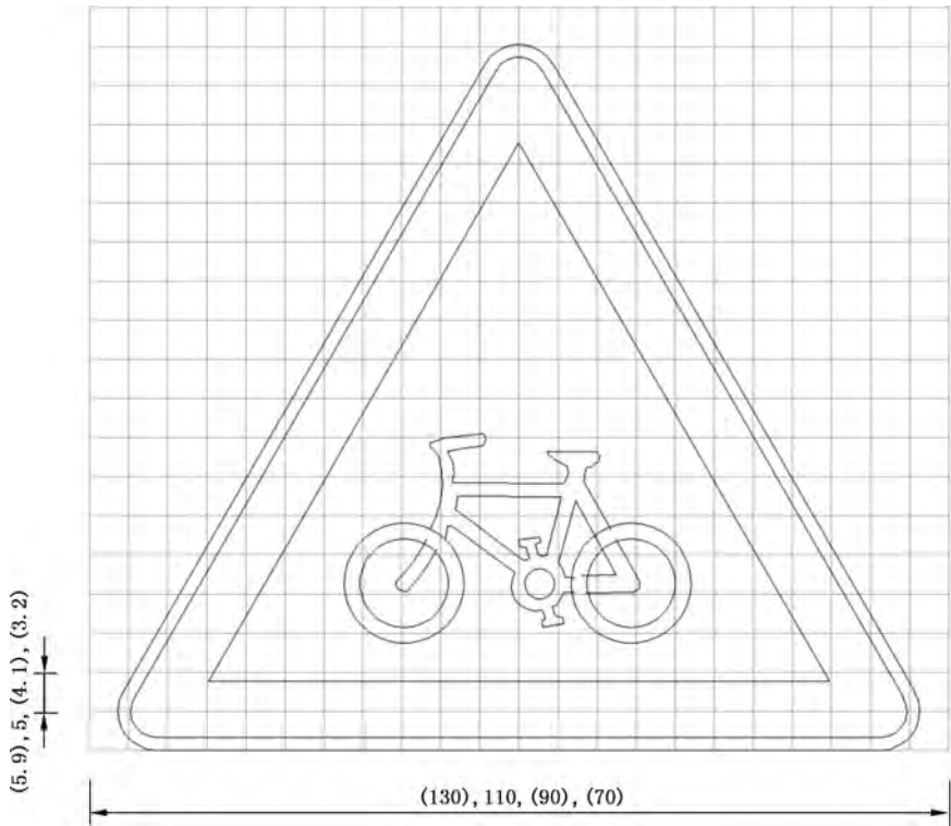
图 E.128 对应警 13 的制作图例
