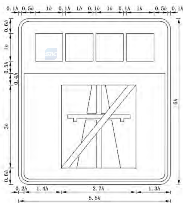
图 E.227 对应路 60 的制作图例
