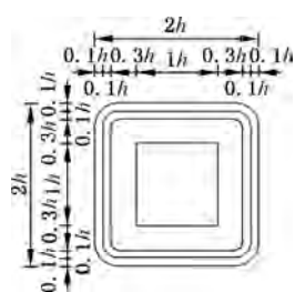
图 E.190 对应路 27 的制作图例
