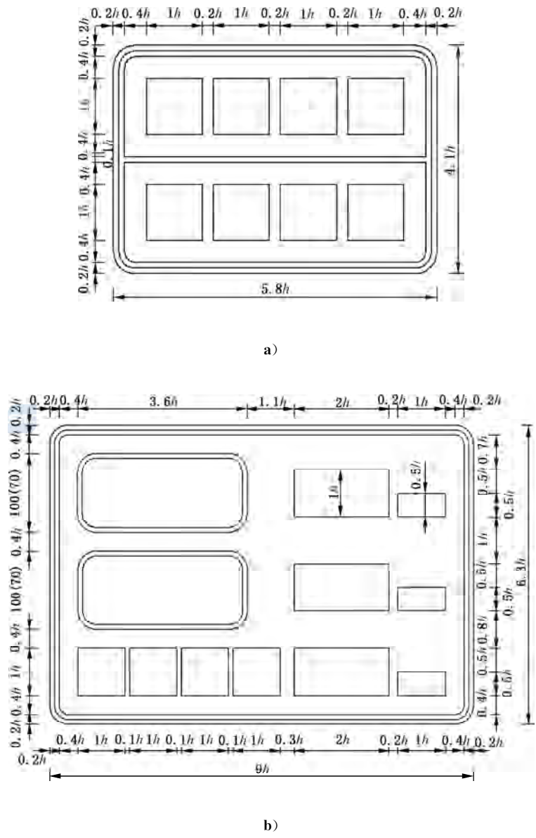
图 E.205 对应路 39 的制作图例
