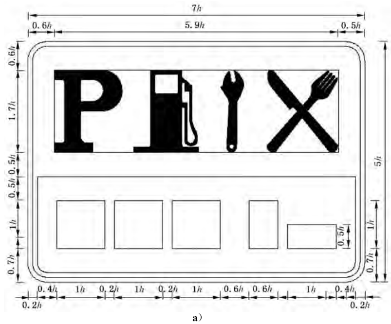
图 E.241 对应路 74 的制作图例
