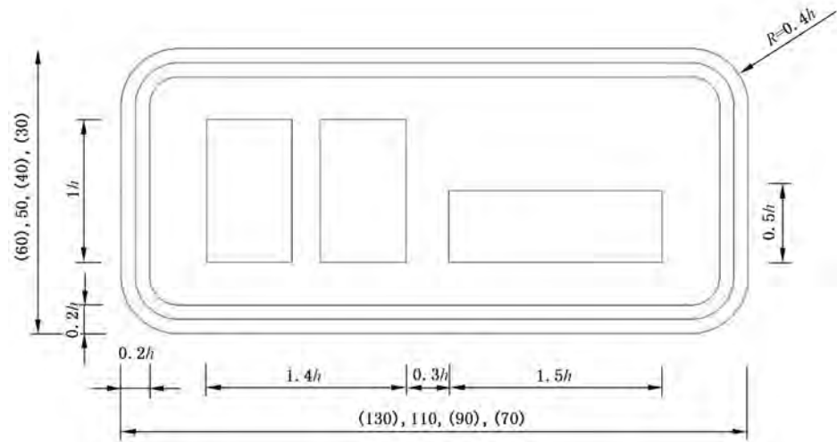
图 E.156 对应警 38 的制作图例
