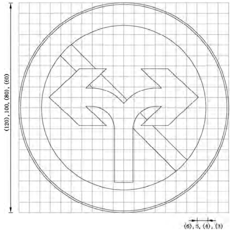
图 E.26 对应禁 26 的制作图例
