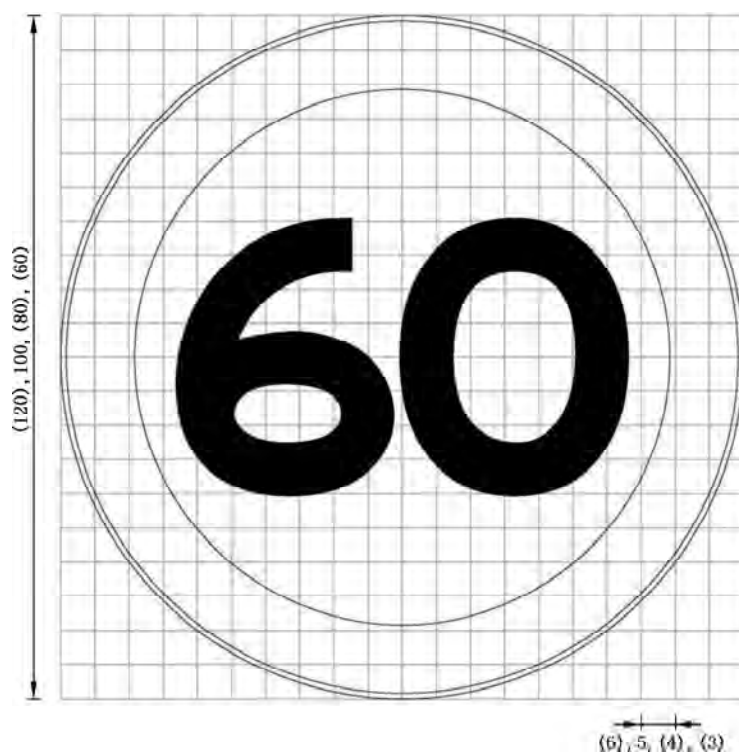
图 E.39 对应禁 39 的制作图例
