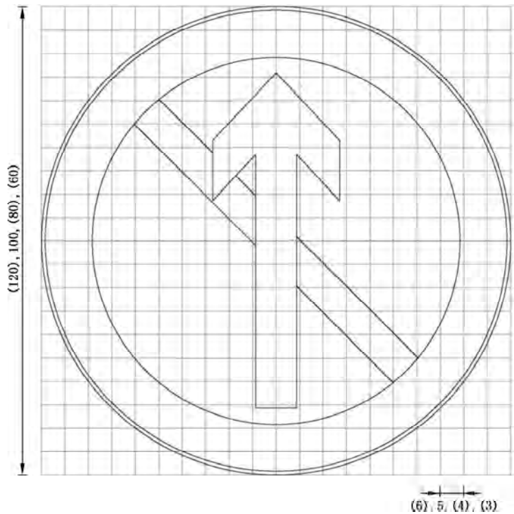
图 E.25 对应禁 25 的制作图例
