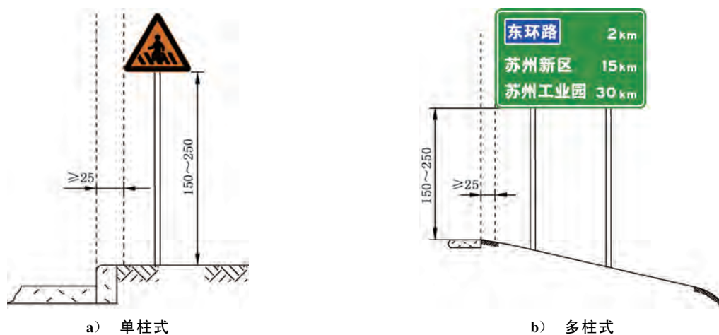
图5 柱式
