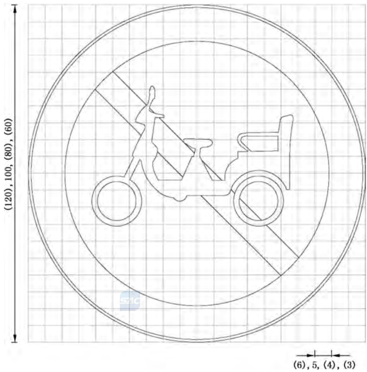
图 E.17 对应禁 17 的制作图例
