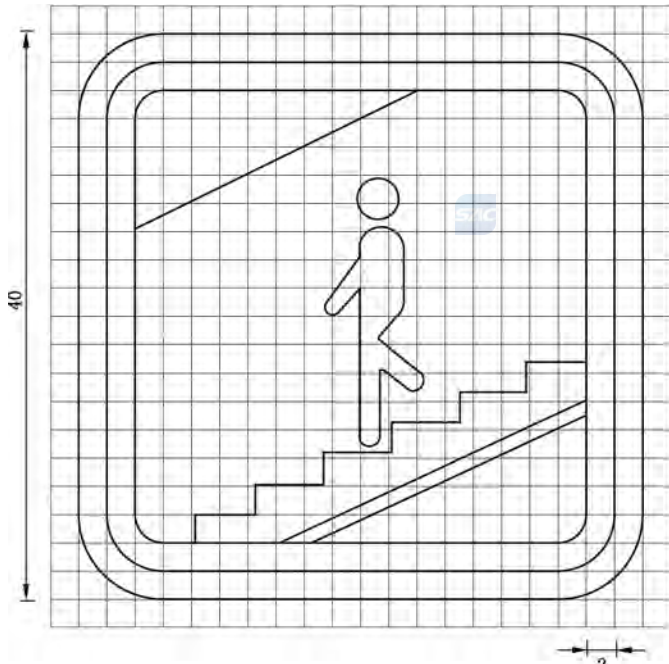
图 E.181 对应路 17 的制作图例
