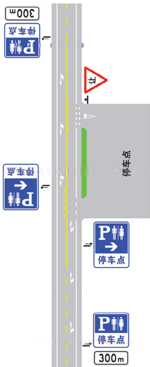
图 H.3 停车点标志设置示例
