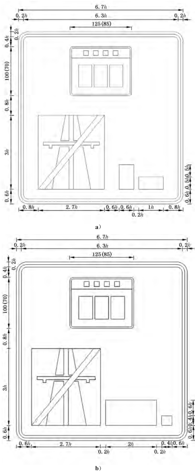
图 E.224 对应路 57 的制作图例
