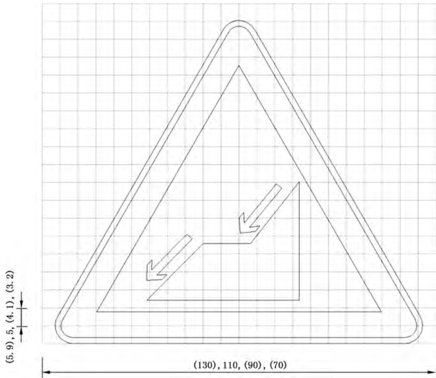
图 E.119 对应警 6 的制作图例
