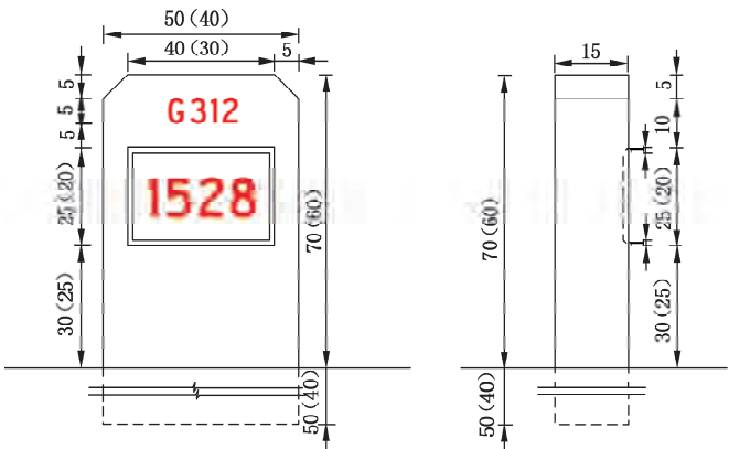
图 243 里程碑
