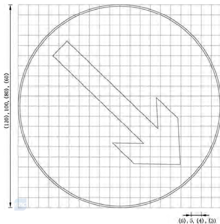
图 E.56 对应示 7 的制作图例
