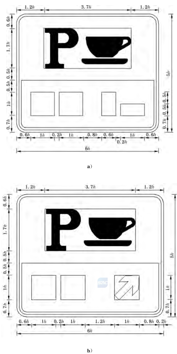
图 E.243 对应路 76 的制作图例
