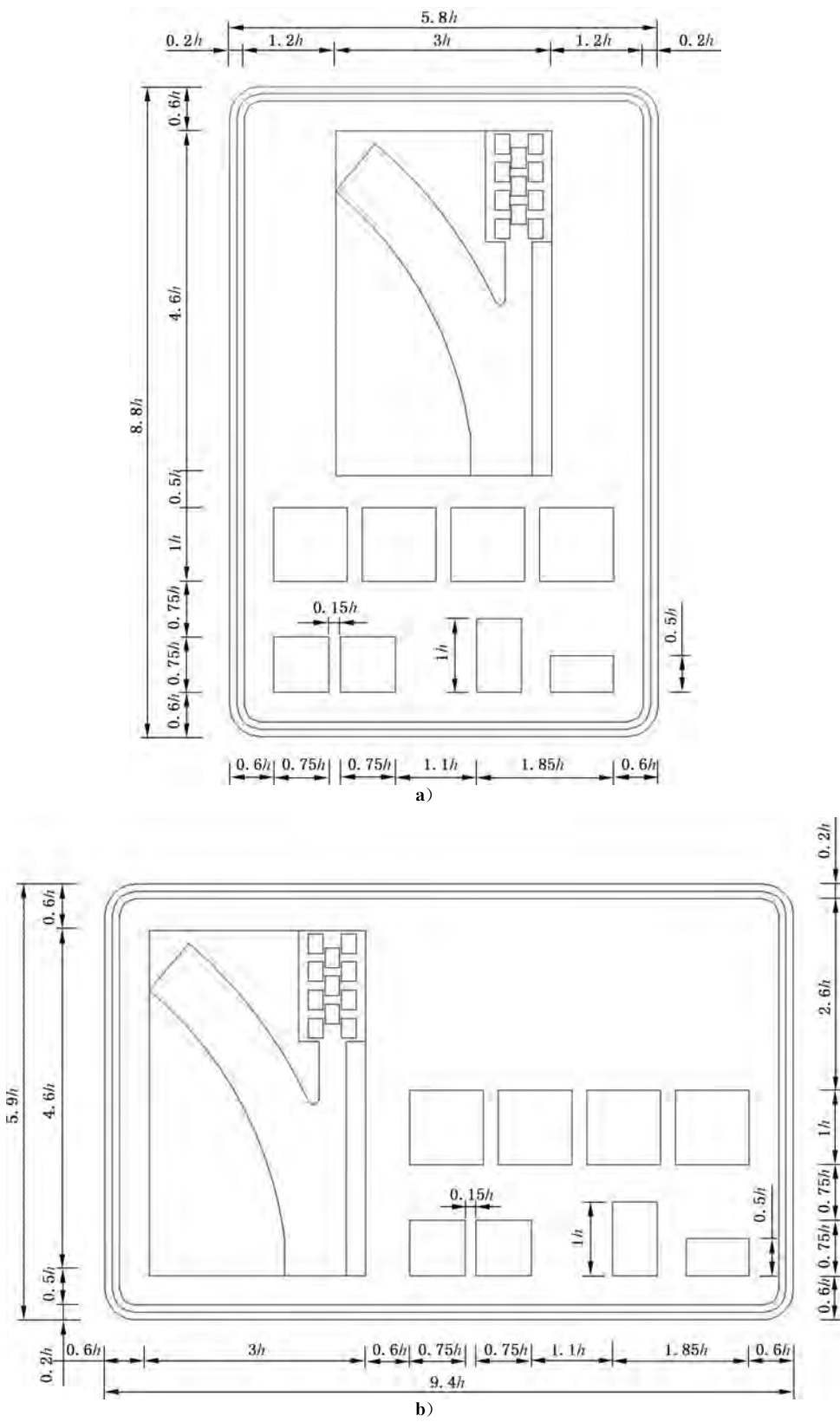
图 E.165 对应避险车道预告标志的制作图例
