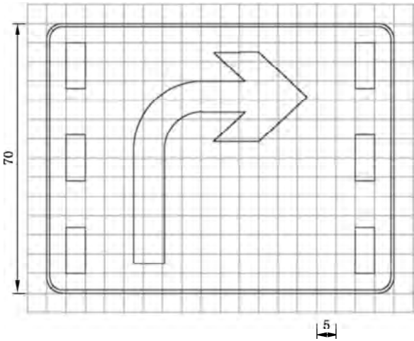
图 E.66 对应示 17 的制作图例
