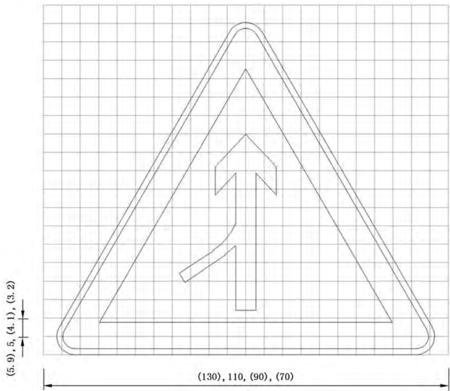
图 E.159 对应警 41-1 的制作图例
