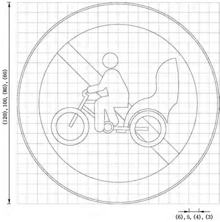
图 E.18 对应禁 18 的制作图例
