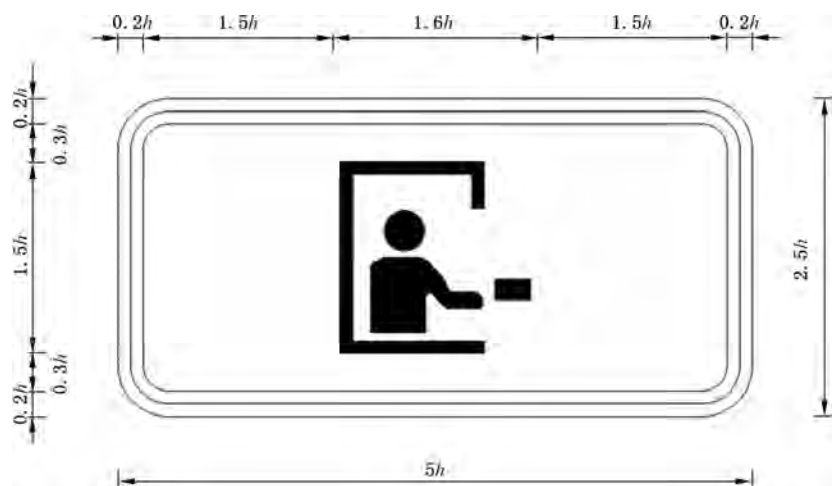
图 E.240 对应路 73 的制作图例
