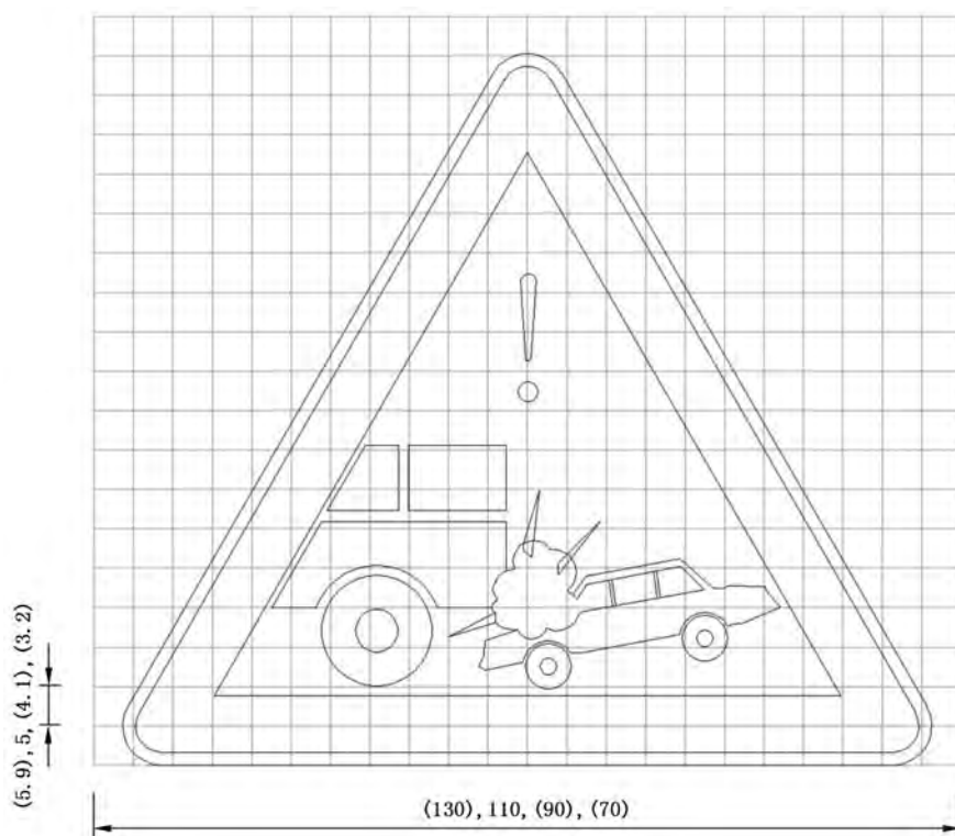
图 E.149 对应警 33 的制作图例
