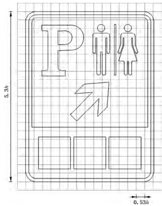
图 E.184 对应路 20 的制作图例
