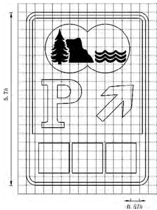
图 E.185 对应路 21 的制作图例
