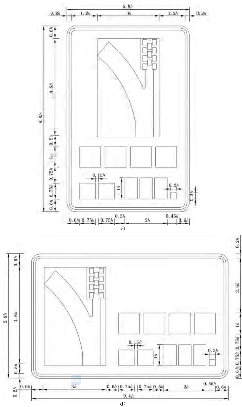
图 E.165 对应避险车道预告标志的制作图例 (续)
