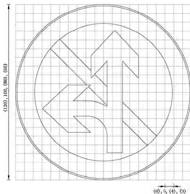
图 E.27 对应禁 27 的制作图例
