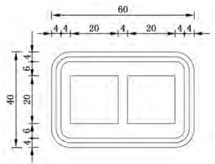
图 E.252 对应辅 14 的制作图例
