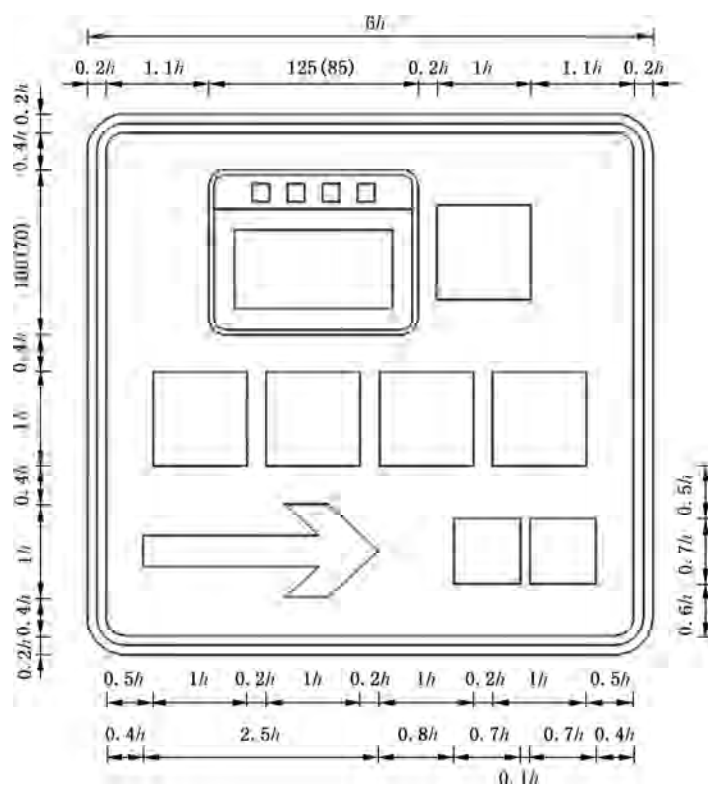
图 E.195 对应路 30 的制作图例(续)
