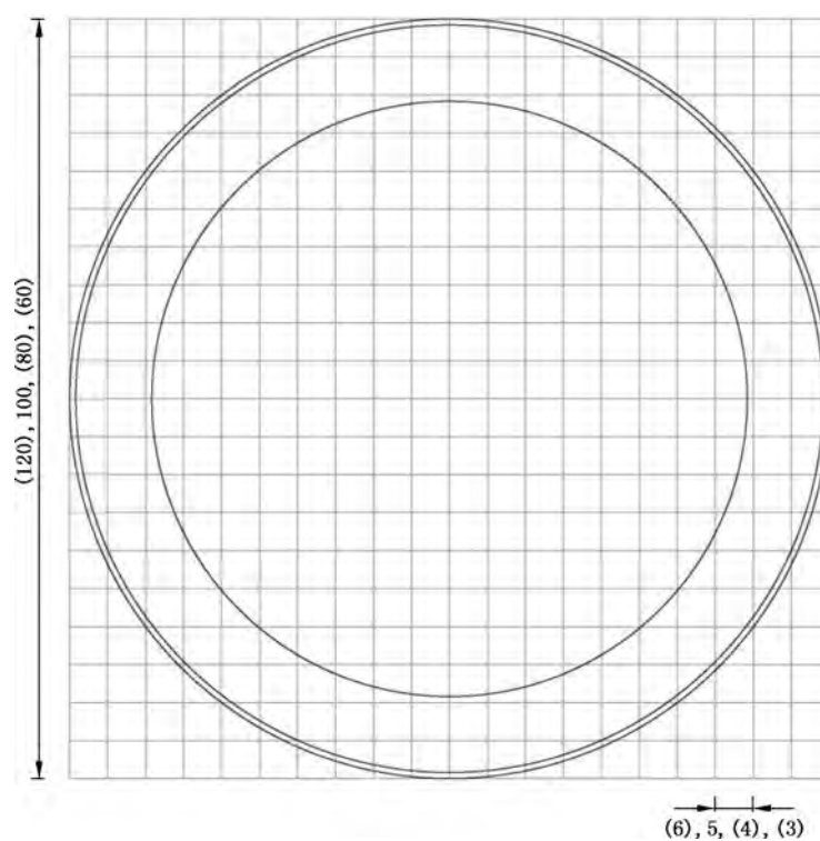
图 E.4 对应禁 4 的制作图例
