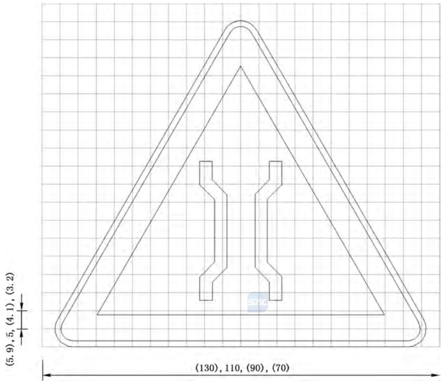
图 E.123 对应警 8 的制作图例
