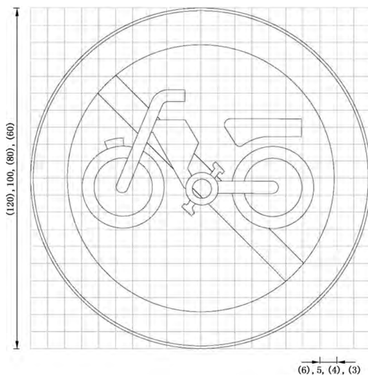
图 E.15 对应禁 15 的制作图例
