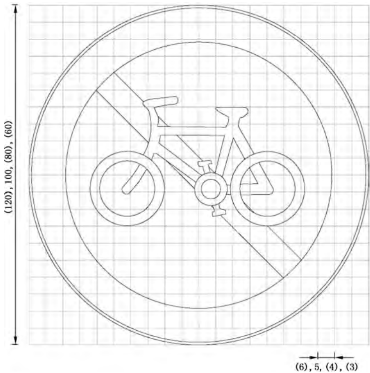
图 E.14 对应禁 14 的制作图例
