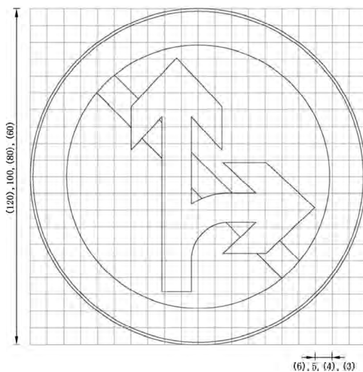
图 E.28 对应禁 28 的制作图例
