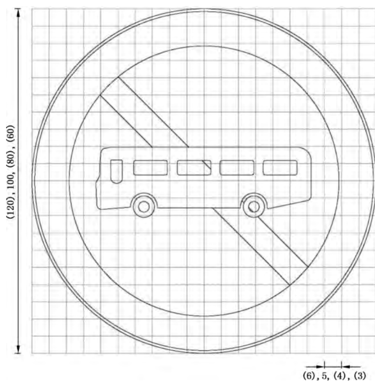
图 E.7 对应禁 7 的制作图例
