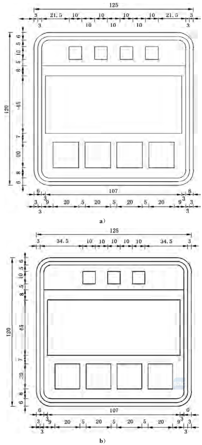
图 E.202 对应路 36 的制作图例
