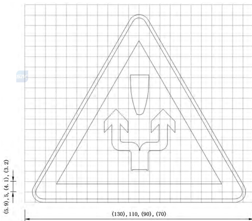
图 E.150 对应警 34-1 的制作图例
