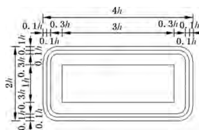
图 E.171 对应路 5 的制作图例
