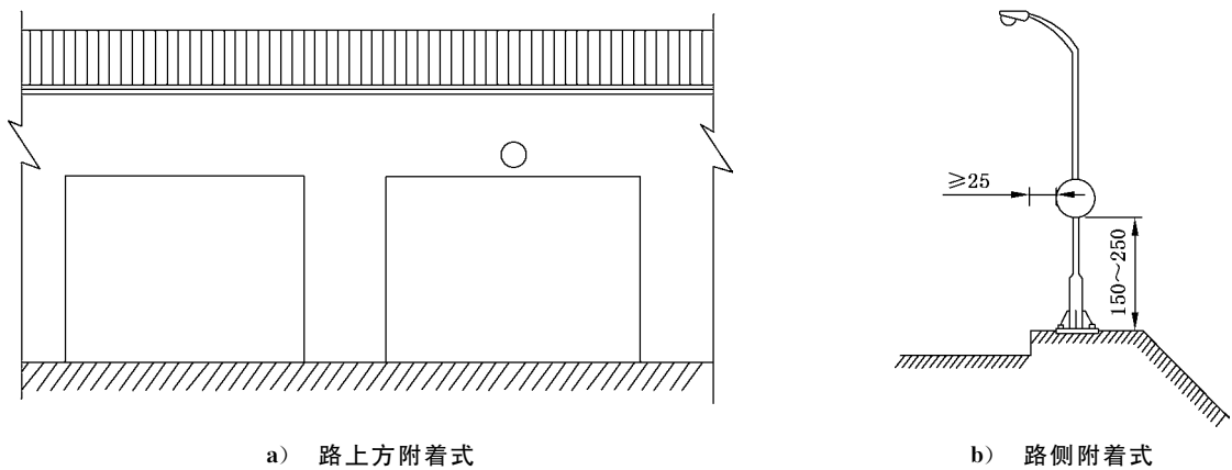
图8 附着式
