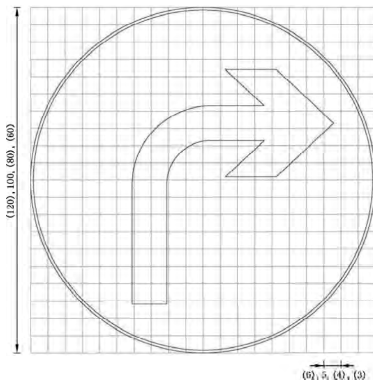
图 E.52 对应示 3 的制作图例
