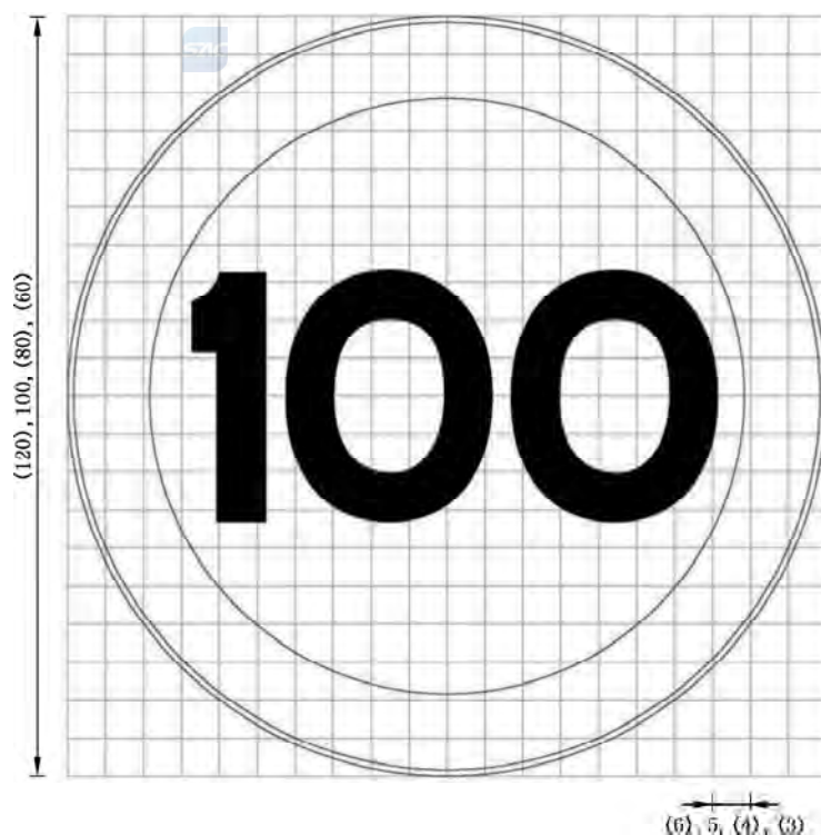
图 E.40 三位数字的限制速度标志制作图例
