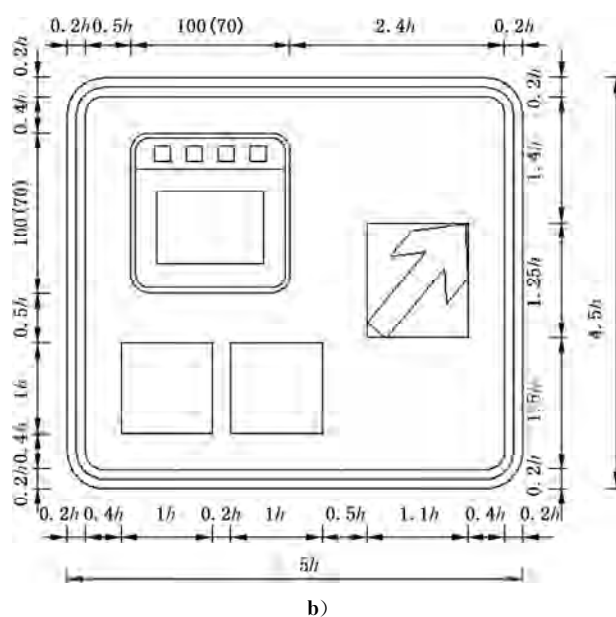
图 E.199 对应路 34 的制作图例
