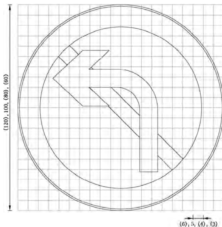
图 E.23 对应禁 23 的制作图例
