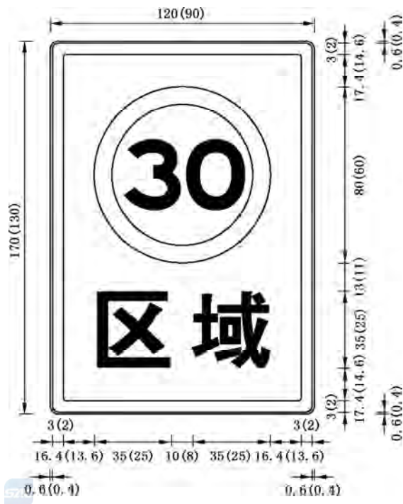
图 E.44 对应禁 43 的制作图例
