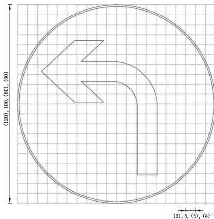
图 E.51 对应示 2 的制作图例
