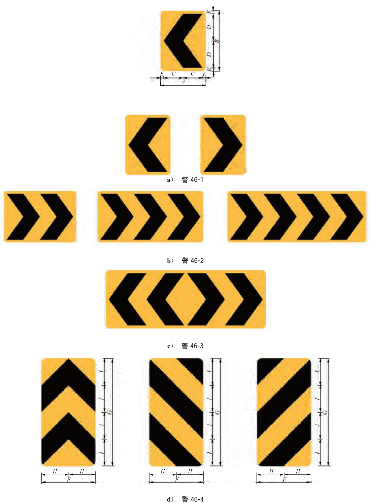
图 199 线形诱导标(警 46)
