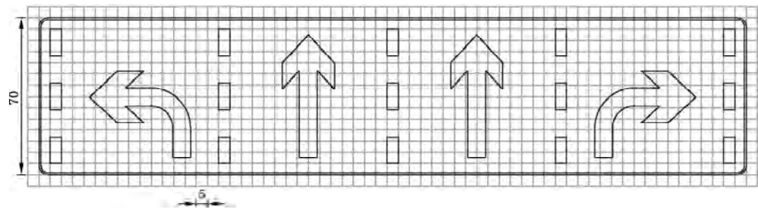
图 E.73 对应组合设置的分向行驶车道标志制作图例
