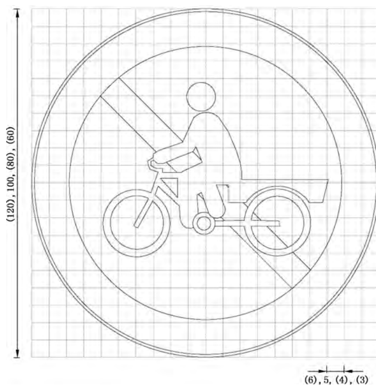
图 E.19 对应禁 19 的制作图例
