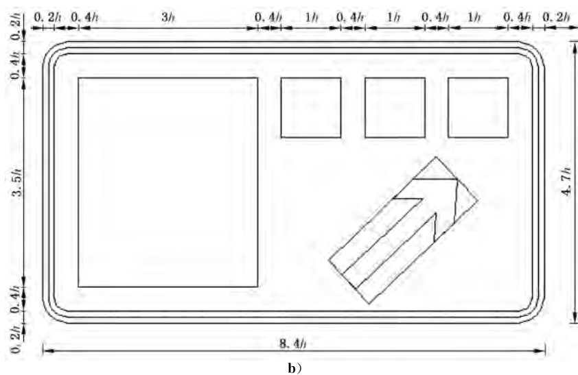
图 E.246 对应旅 2 的制作图例
