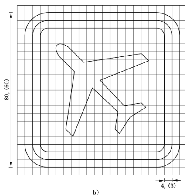
图 E.176 对应路 12 的制作图例
