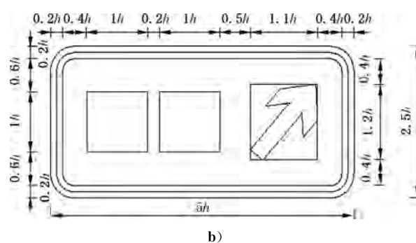
图 E.198 对应路 33 的制作图例(续)
