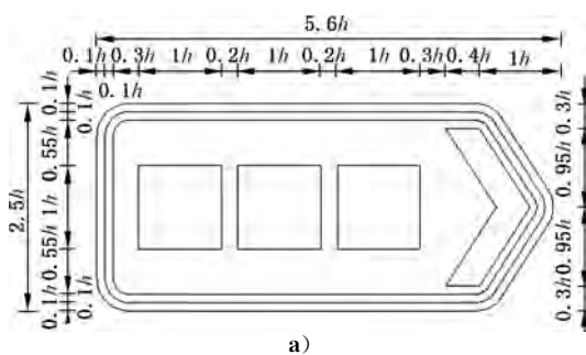
图 E.172 对应路 6、路 9、路 10 的制作图例
