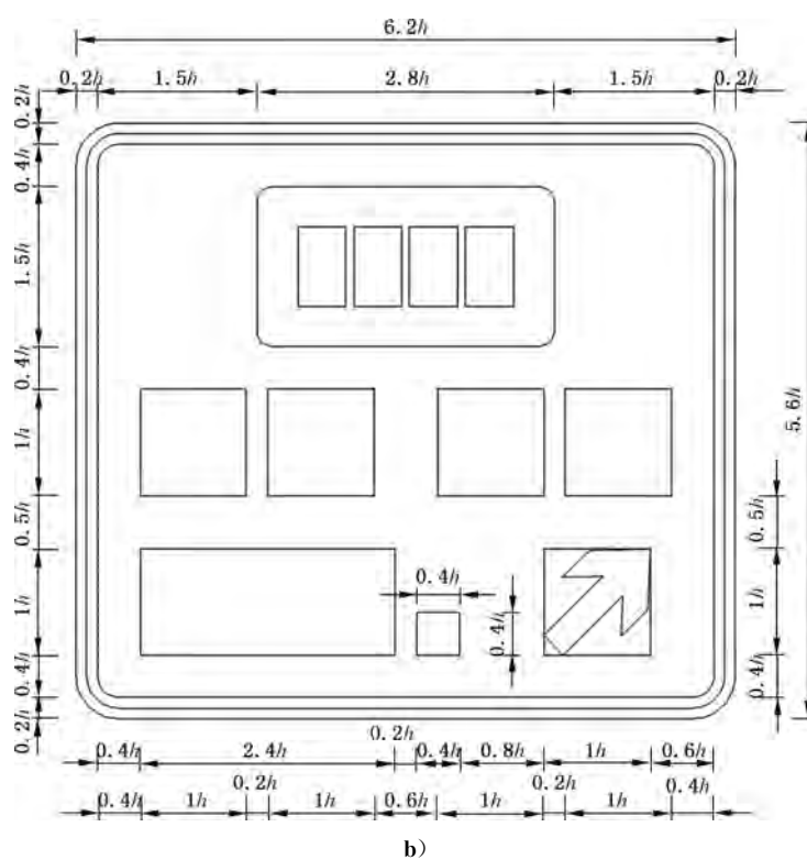
图 E.208 对应路 42 的制作图例
