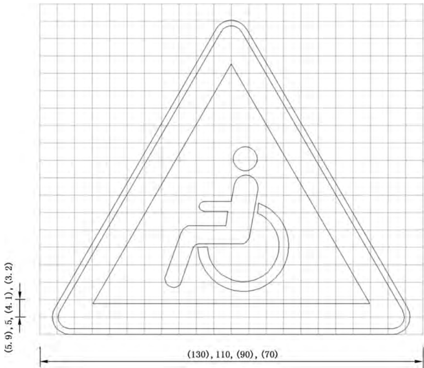
图 E.127 对应警 12 的制作图例
