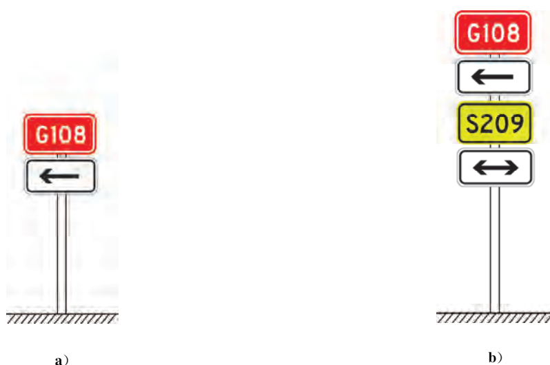
图 209 预告前方交叉道路编号的预告标志示例
