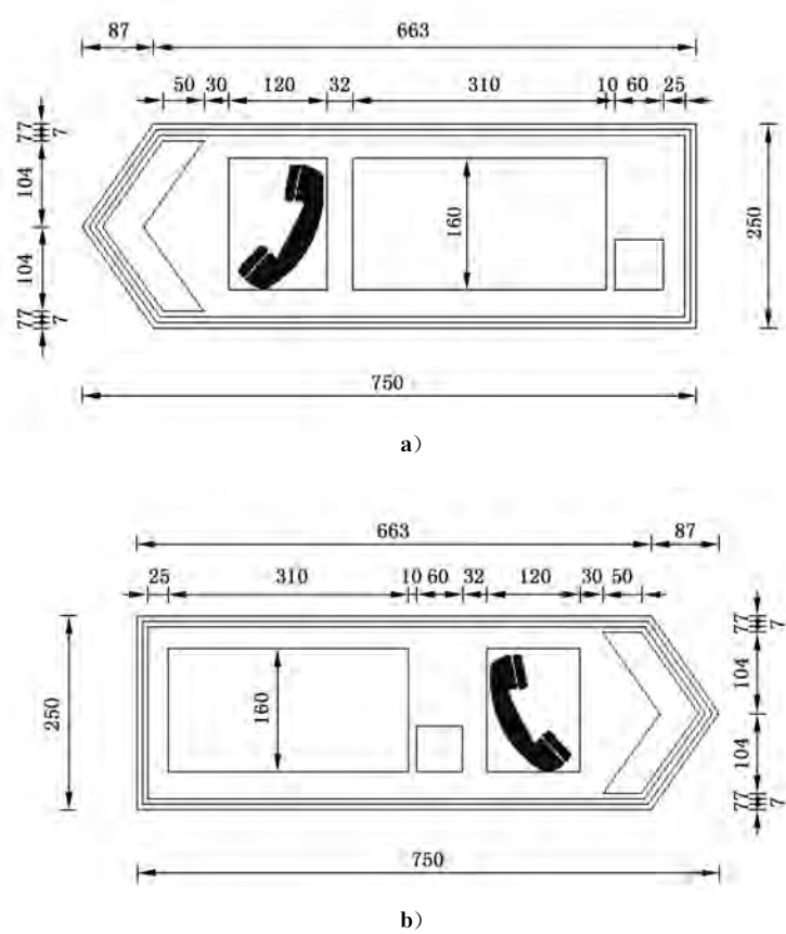
图 E.235 对应路 68 的制作图例
