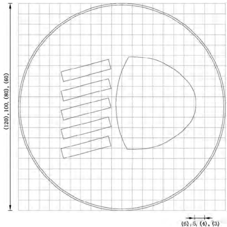
图 E.62 对应示 13 的制作图例
