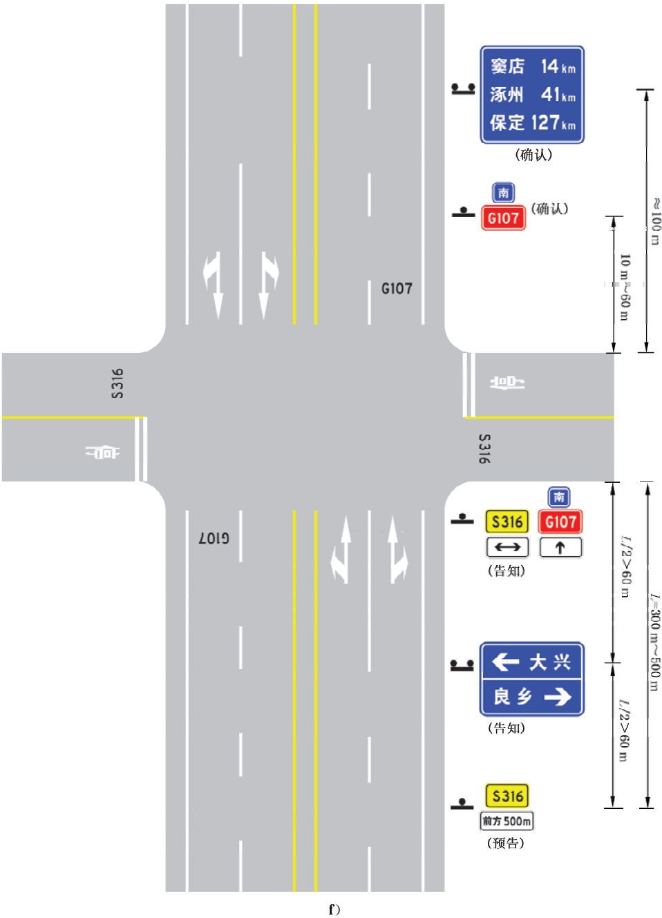
图 H.2 公路交叉口指路标志设置示例 (续)
