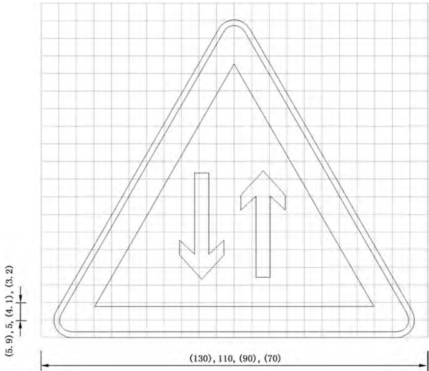
图 E.124 对应警 9 的制作图例
