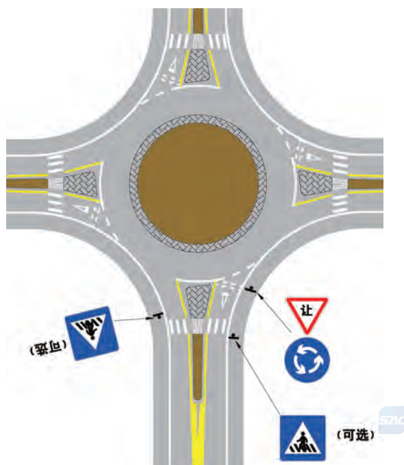
图 89 环岛行驶标志设置示例
