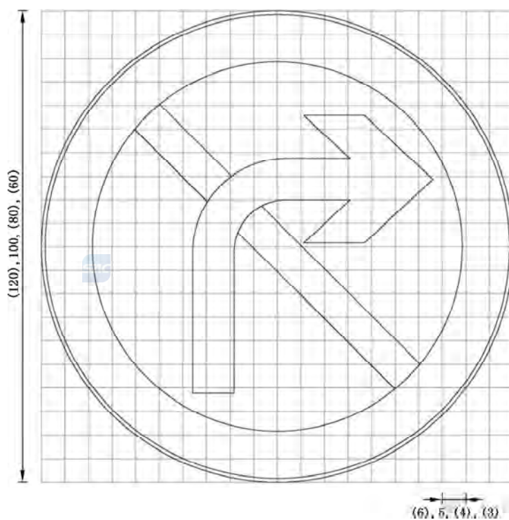
图 E.24 对应禁 24 的制作图例
