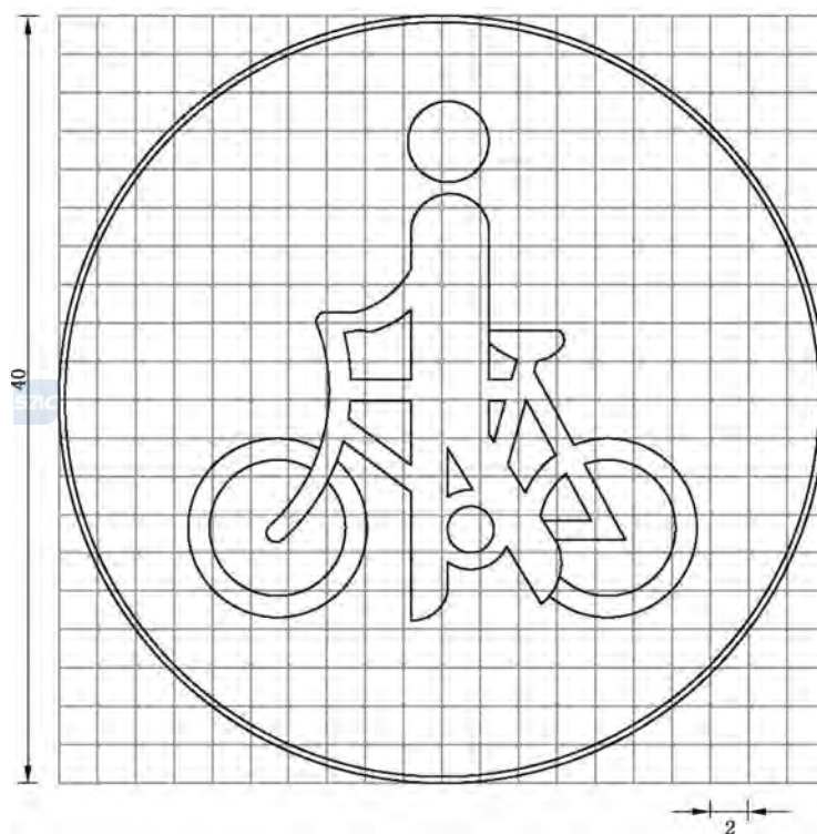
图 E.89 对应示 38 的制作图例
