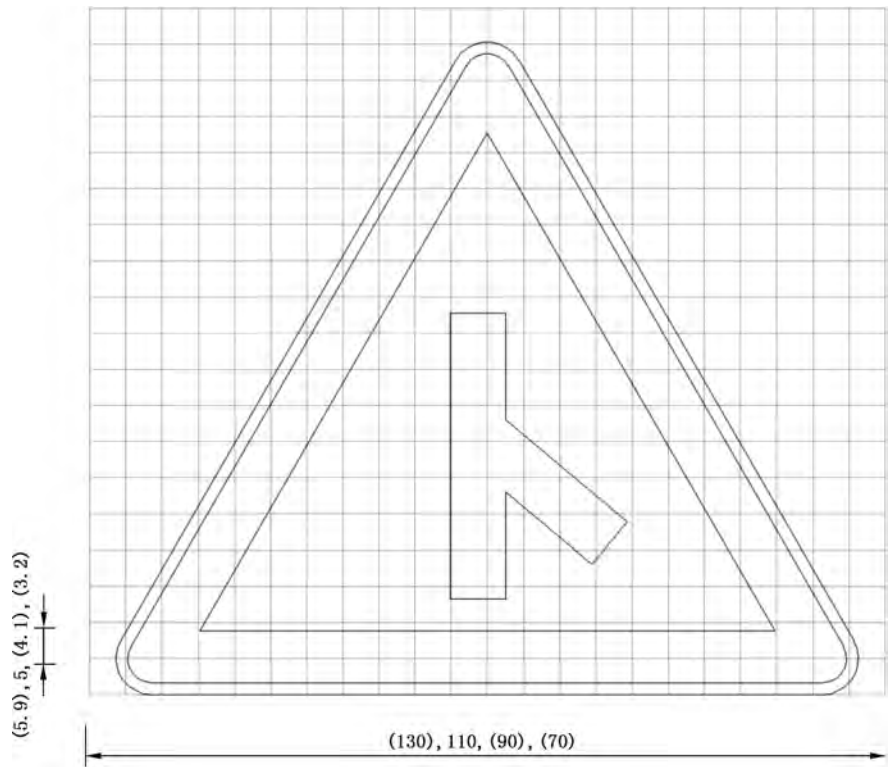
图 E.103 对应警 1-4 的制作图例
