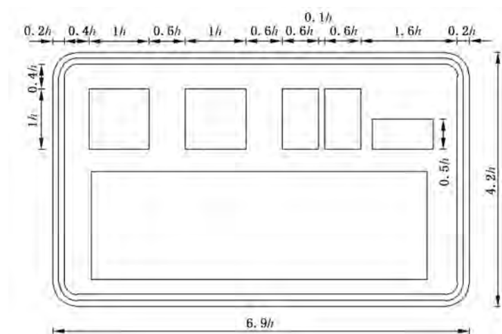
图 E.245 对应旅 1 的制作图例
