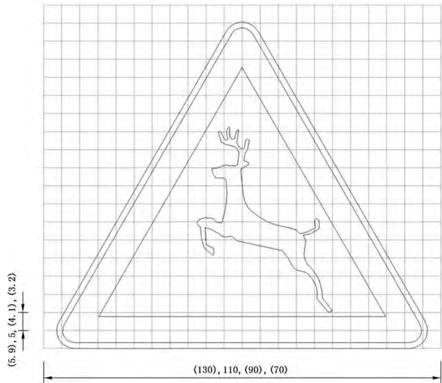
图 E.131 对应警 16 的制作图例
