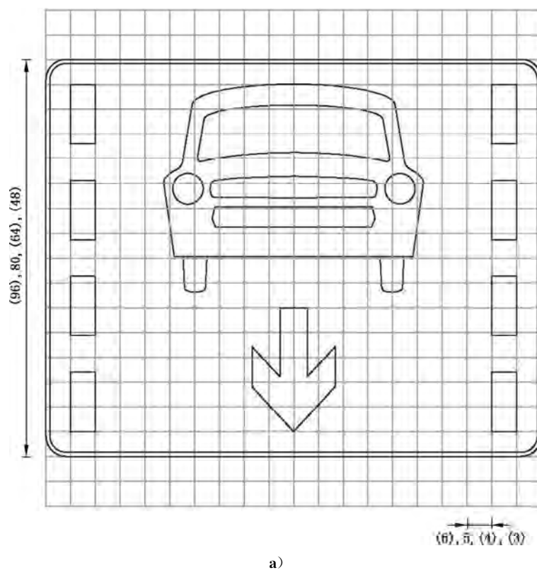
图 E.75 对应示 25 的制作图例
