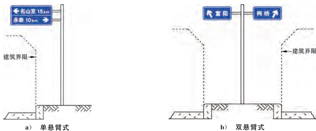
图6 悬臂式
