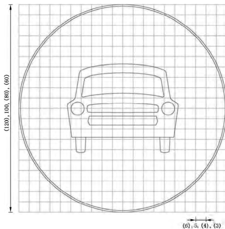
图 E.74 对应示 24 的制作图例
