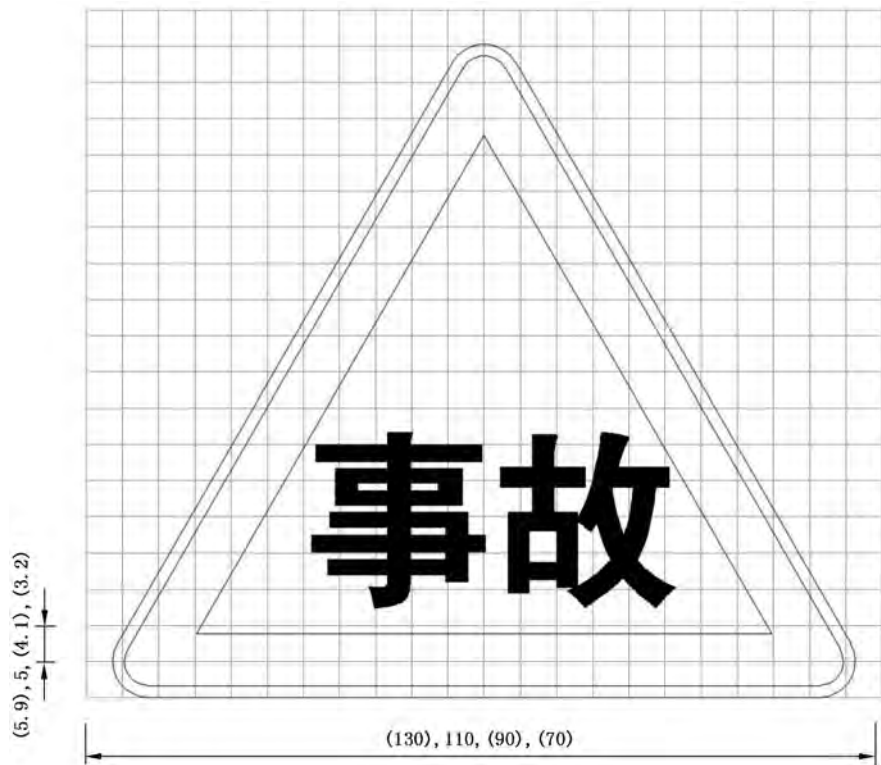
图 E.155 对应警 37 的制作图例
