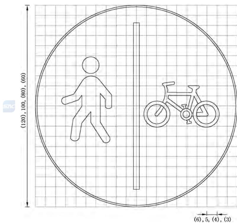
图 E.86 对应示 36-1 的制作图例
