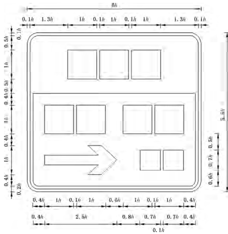
图 E.196 对应路 31 的制作图例 (续)
