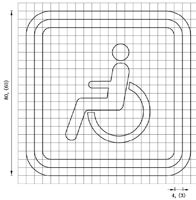
图 E.182 对应路 18 的制作图例
