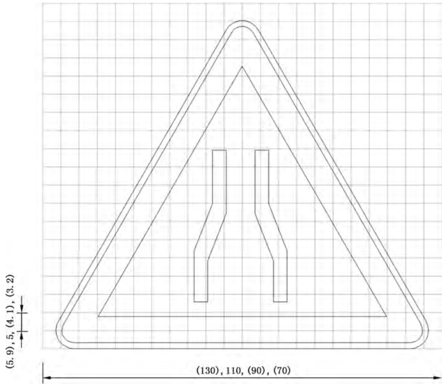
图 E.120 对应警 7-1 的制作图例
