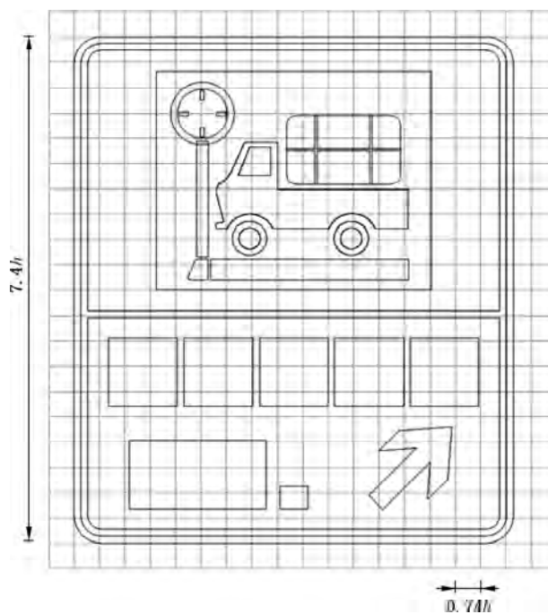
图 E.187 对应路 23 的制作图例
