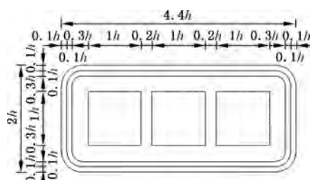
图 E.171 对应路 5 的制作图例
