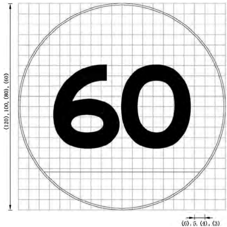
图 E.63 对应示 14 的制作图例
