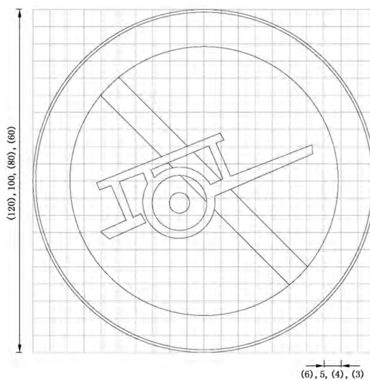
图 E.20 对应禁 20 的制作图例
