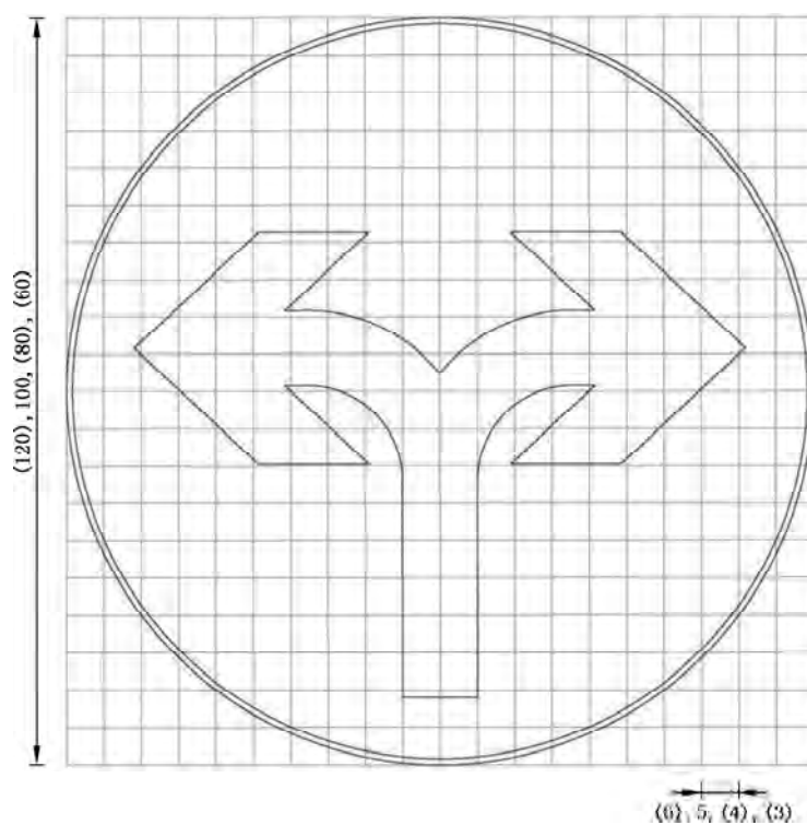
图 E.55 对应示 6 的制作图例
