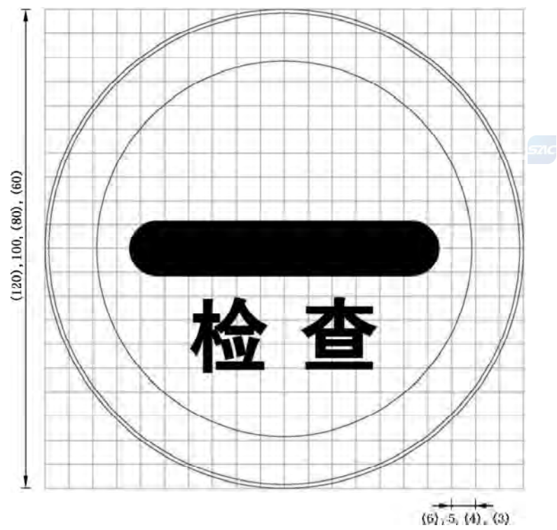
图 E.42 对应禁 41 的制作图例
