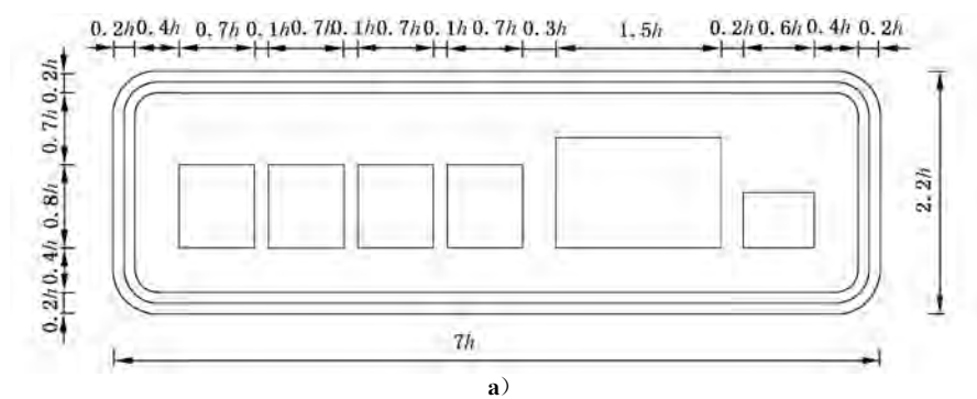
图 E.221 对应路 54 的制作图例
