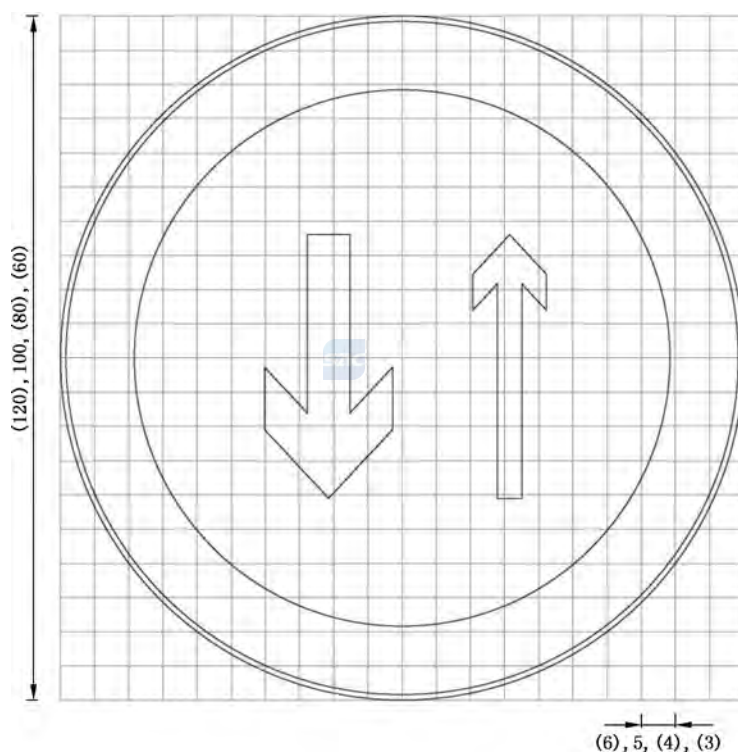
图 E.3 对应禁 3 的制作图例
