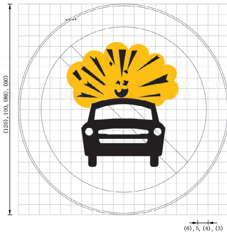
图 E.43 对应禁 42 的制作图例
