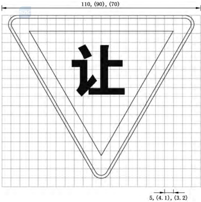
图 E.2 对应禁 2 的制作图例
