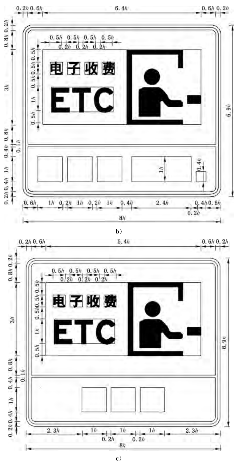
图 E.237 对应路 70 的制作图例 (续)
