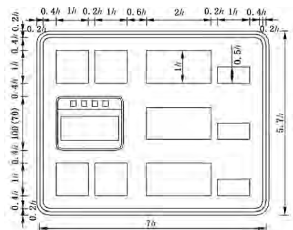
图 E.204 对应路 38 的制作图例
