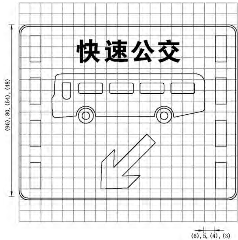
图 E.78 对应示 28 的制作图例
