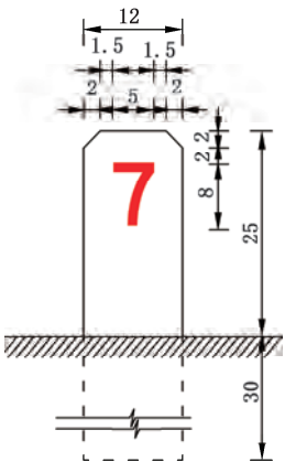
图 245 百米桩
