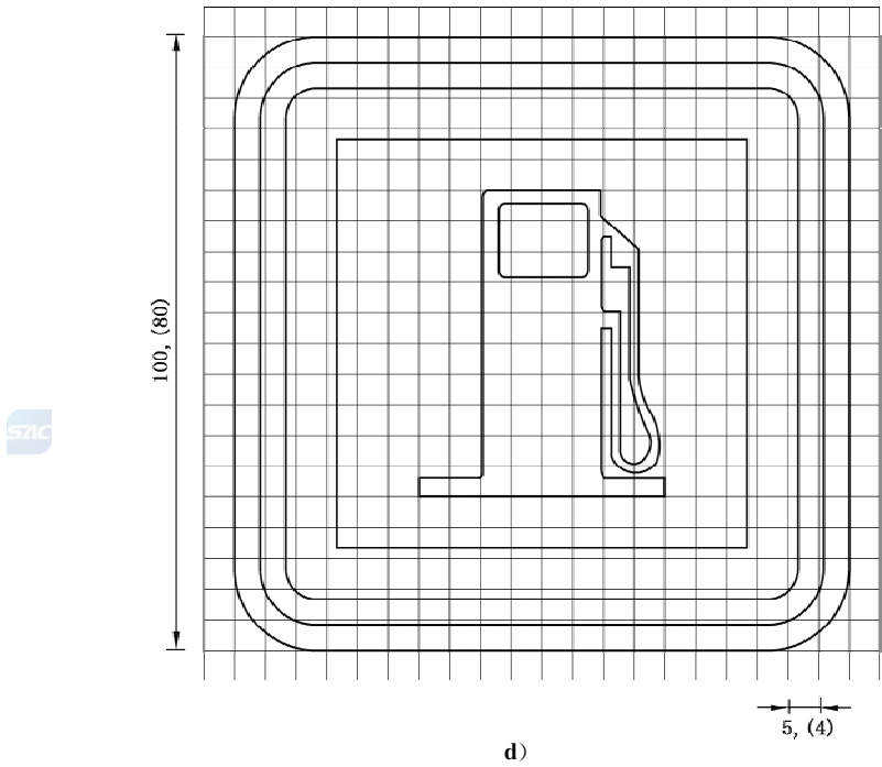
图 E.176 对应路 12 的制作图例（续）
