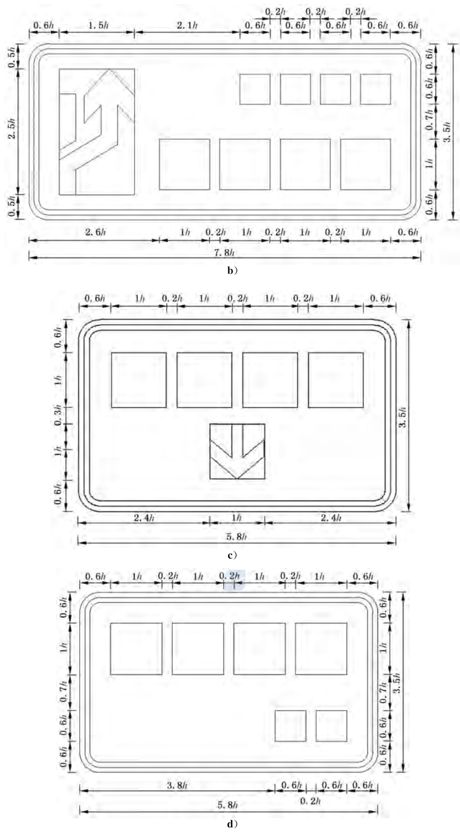
图 E.244 对应路 77 的制作图例 (续)
